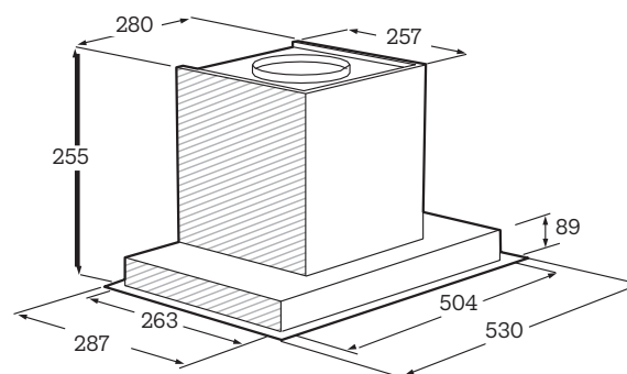
GROUPE FILTRANT 60 cm SOHG1630B
